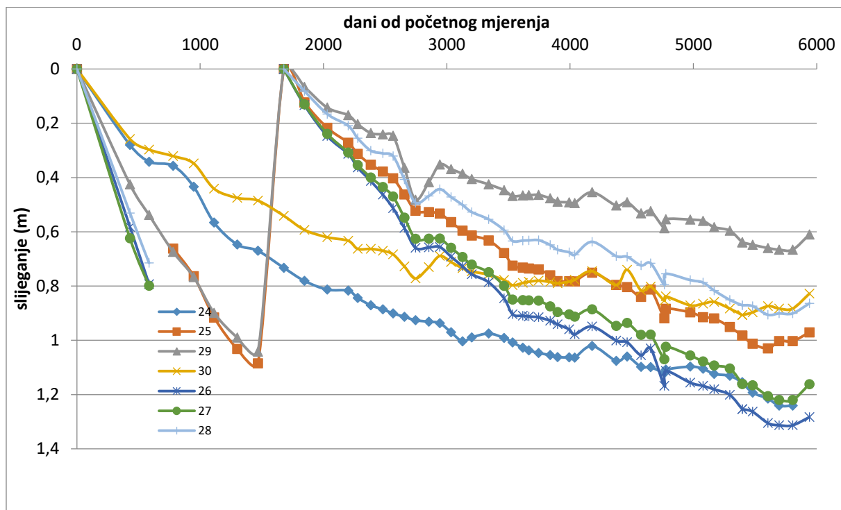
Slika 4. Prikaz konsolidacije repera broj 24, 25, 26, 27, 28, 29, 30. (profil 8). Horizontalna os prikazuje vrijeme u danima a vertikalna os prikazuje slijeganje u metrima. Vrijeme je prikazano u linearnom mjerilu. Početni datum mjerenja slijeganja je 24.11.2006. a nakon obnove repera 30.06.2011, osim repera 24 i 30.
