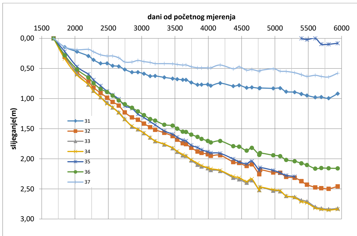
Slika 5. Prikaz konsolidacije repera broj 31, 32, 34, 35, 36, 37 (profil 10). Horizontalna os prikazuje vrijeme u danima a vertikalna os prikazuje slijezanje u metrima. Vrijeme je prikazano u linearnom mjerilu. Početni datum mjerenja slijezanja je 30.06.2011.
