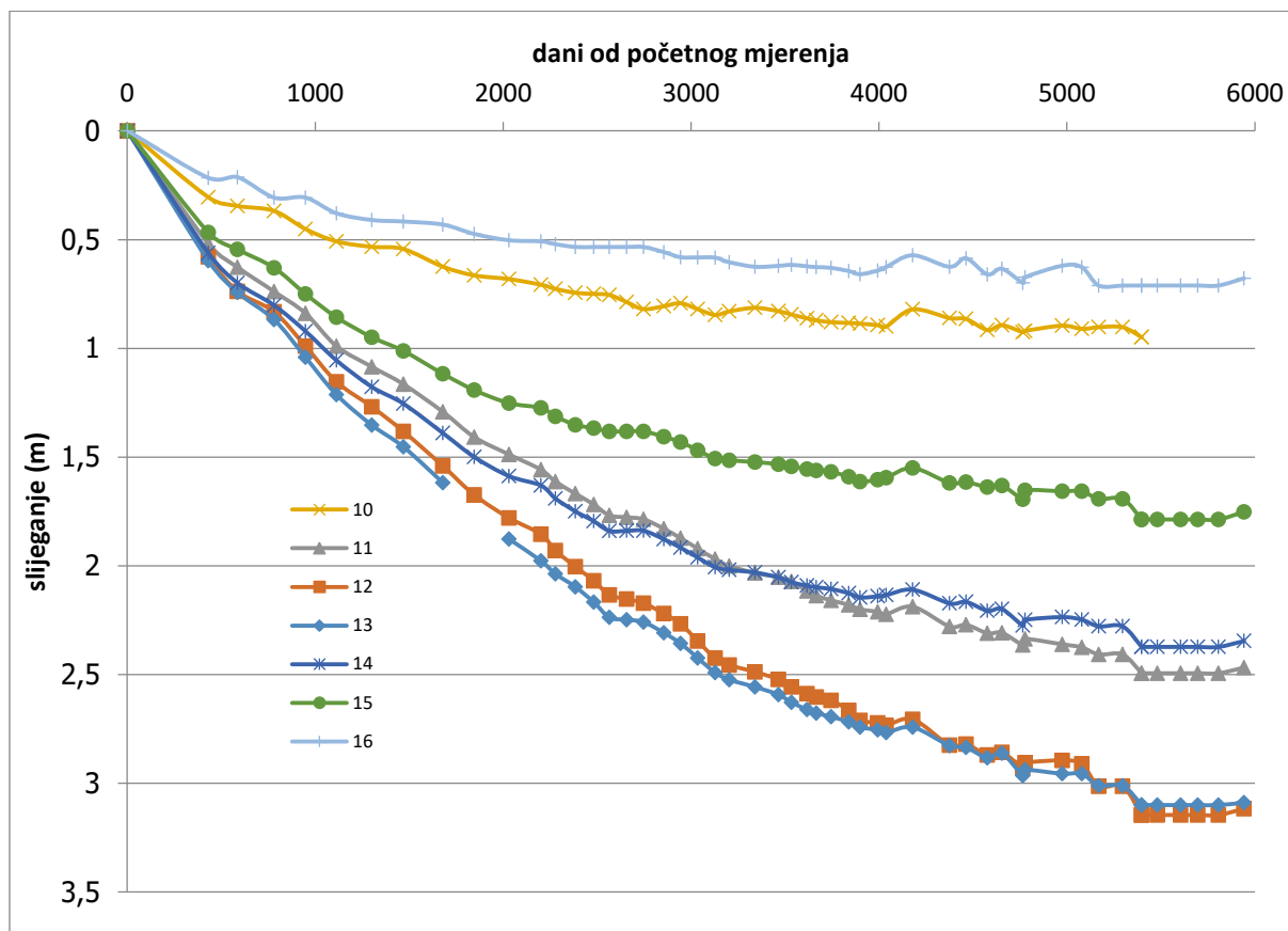
Slika 2. Prikaz konsolidacije repera broj 10, 11, 12, 13, 14, 15, 16 (profil 4). Horizontalna os prikazuje vrijeme u danima a vertikalna os prikazuje slijeganje u metrima. Vrijeme je prikazano u linearnom mjerilu. Početni datum mjerenja slijeganja je 24.11.2006.
