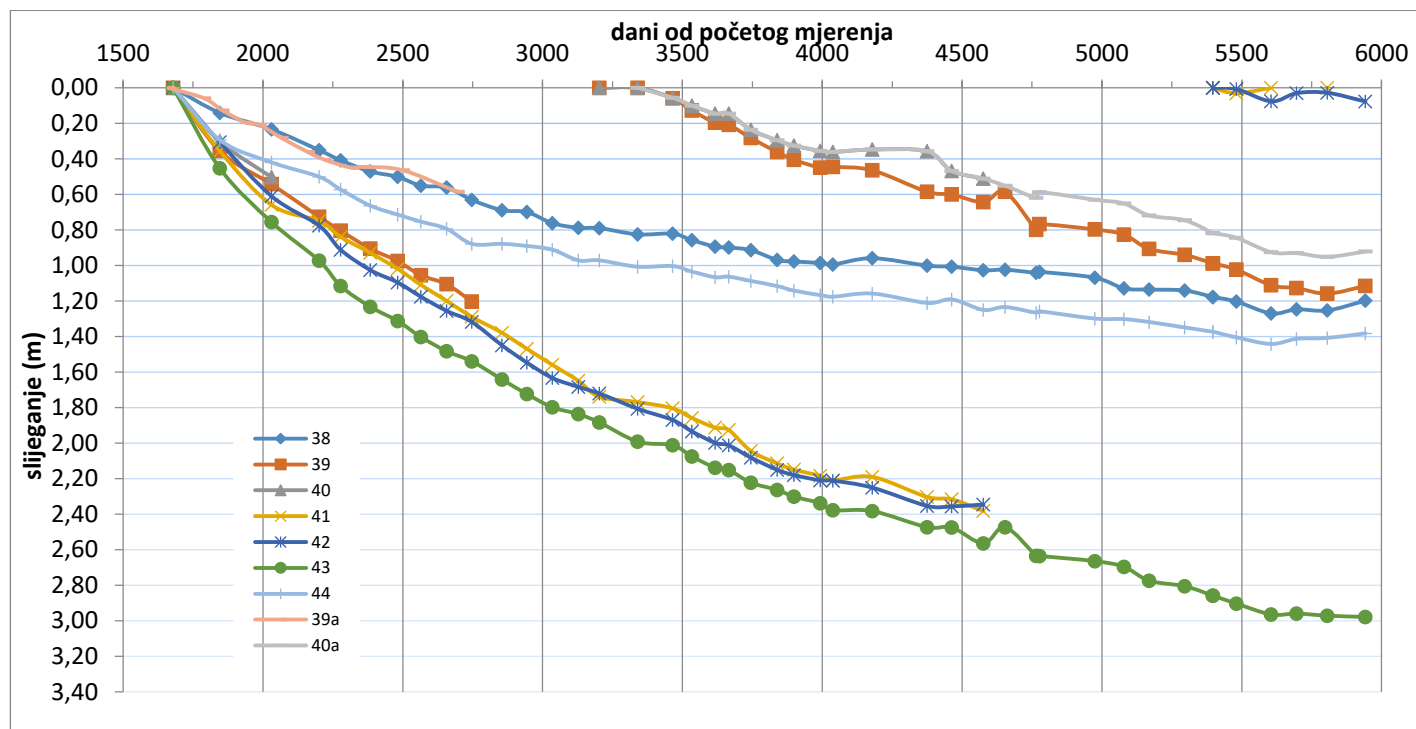
Slika 6. Prikaz konsolidacije repera broj 38, 39, 40, 41, 42, 43, 44 (profil 12). Horizontalna os prikazuje vrijeme u danima, a vertikalna os prikazuje slijezanje u metrima. Vrijeme je prikazano u linearnom mjerilu. Početni datum mjerenja slijezanja je 30.06.2011. Početni datum mjerenja slijezanja repera br. 42 je 03.09.2021.
